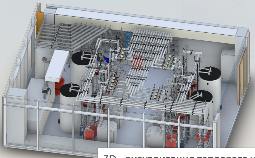
3D - визуализация теплового узла
