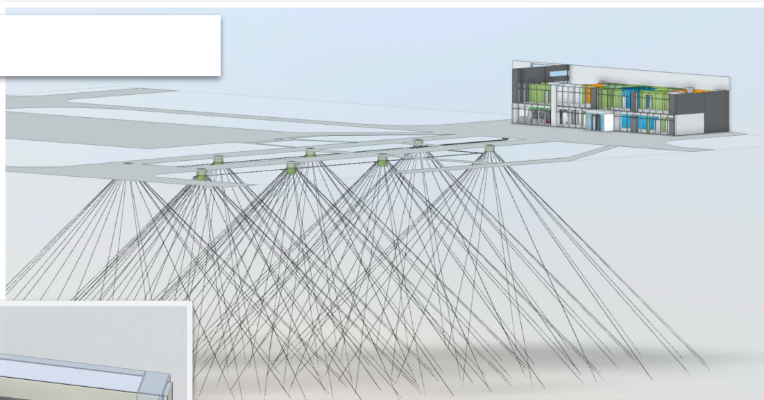
3D - визуализация грунтового теплообменника
